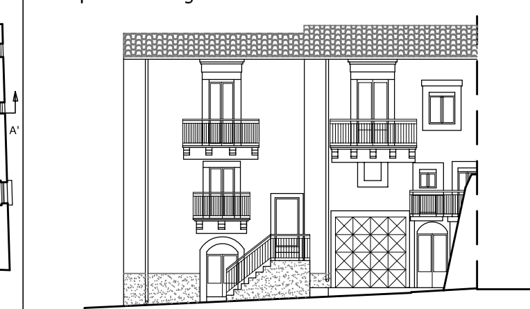
Prospetto su largo Archimede
