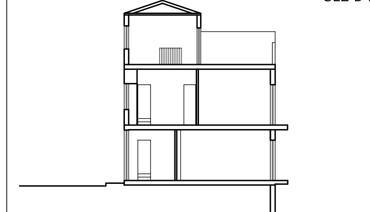
SEZ A-A'
