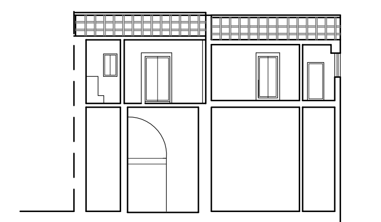
Prospetto su cortile Canova
