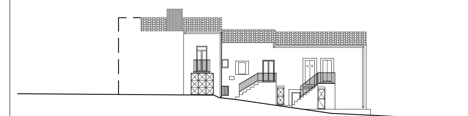
Prospetto su via Garibaldi
